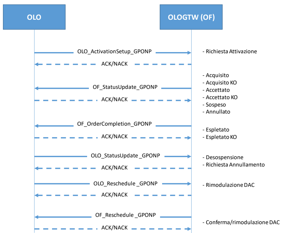
Figura 1: Attivazione servizio GPONP
